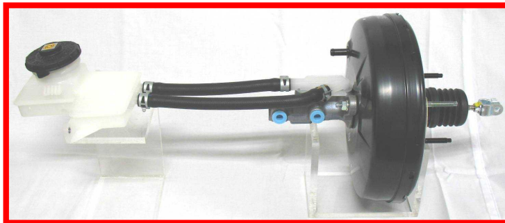
ブランチャー型マスタシリンダ & マスターパワー
